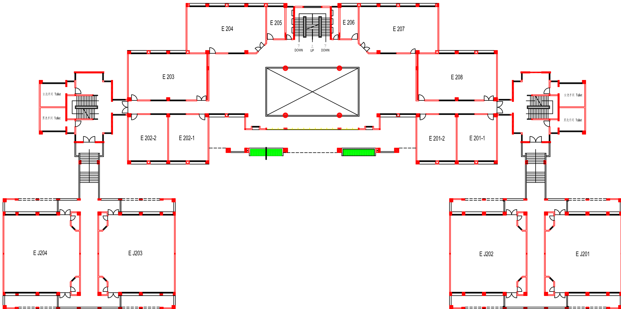
二层平面布置图 2nd Floor Layout
