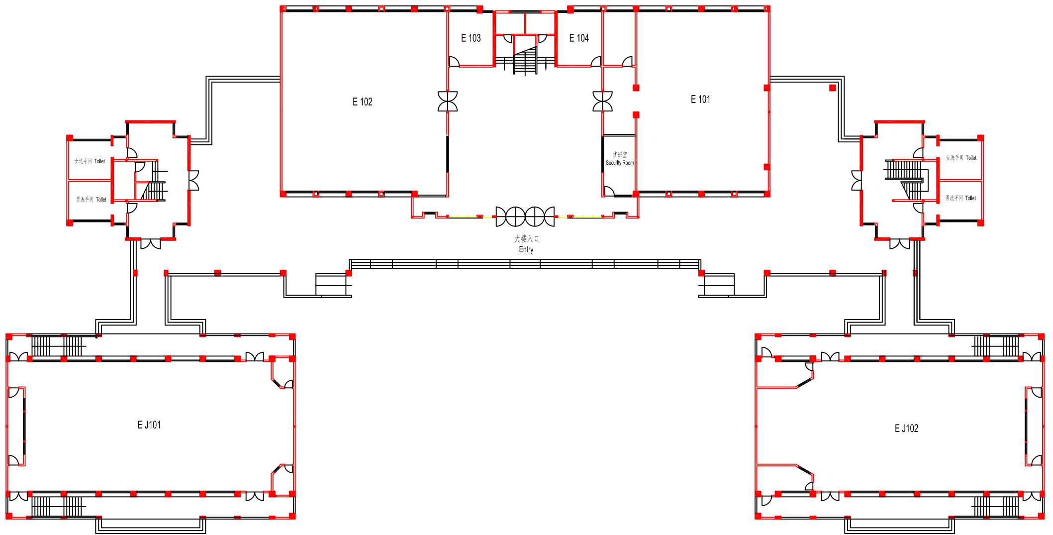
一层平面布置图 1st Floor Layout
