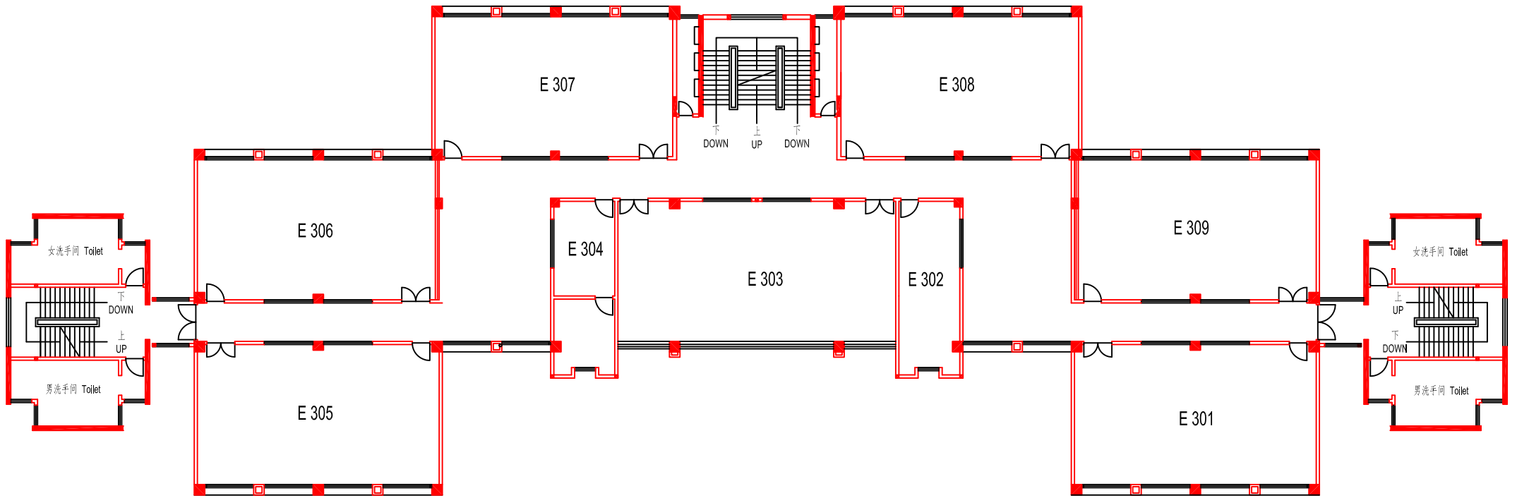
三层平面布置图 3rd Floor Layout
